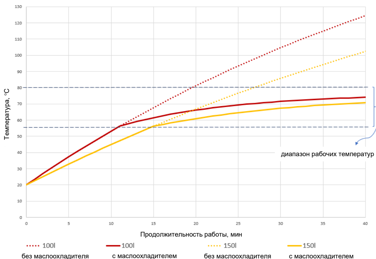
Диаграмма повышения температуры с маслоохладителем и без него
