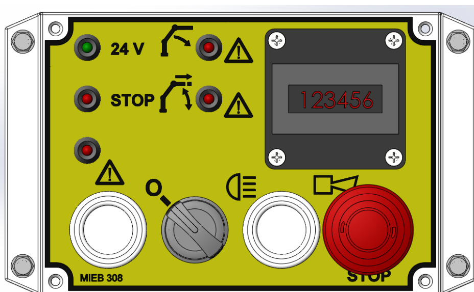
Рис.6: Блок индикации (пример)
