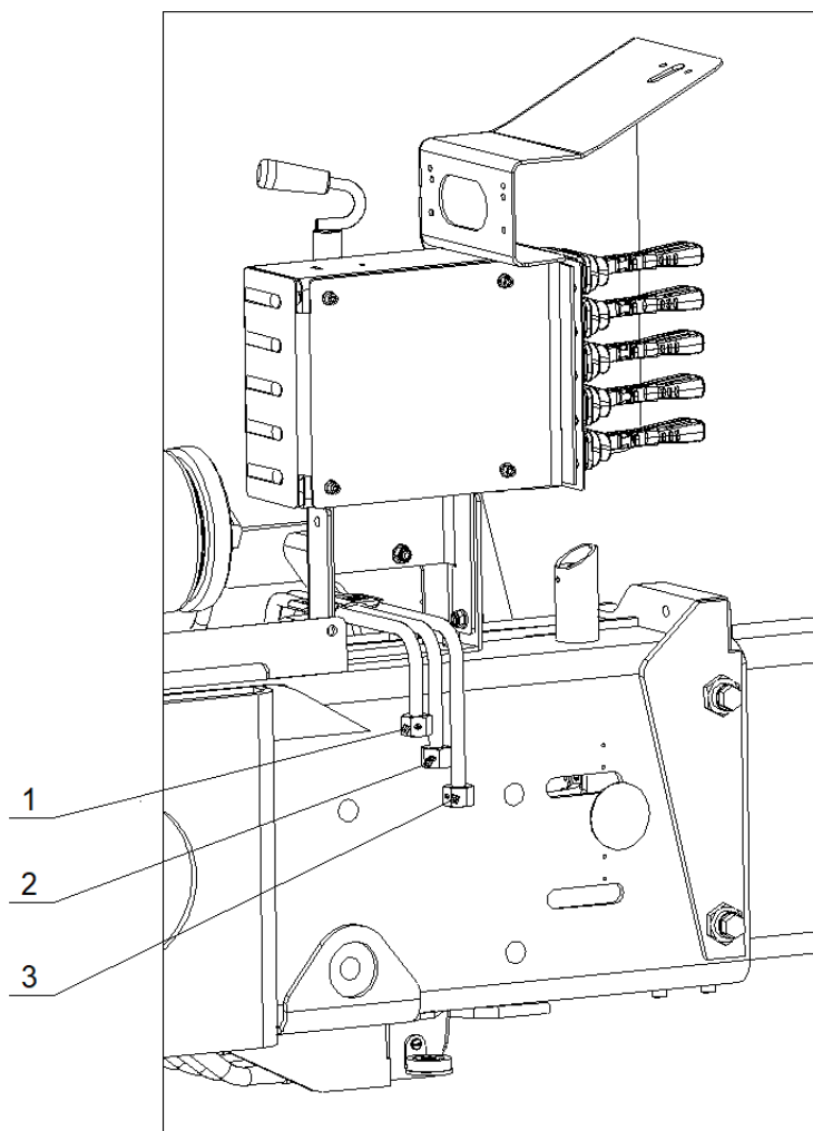
Рис.18: Расположение гидравлических трубок для подключения дополнительных опор на КУ модели ИМ 175Т (пример)
