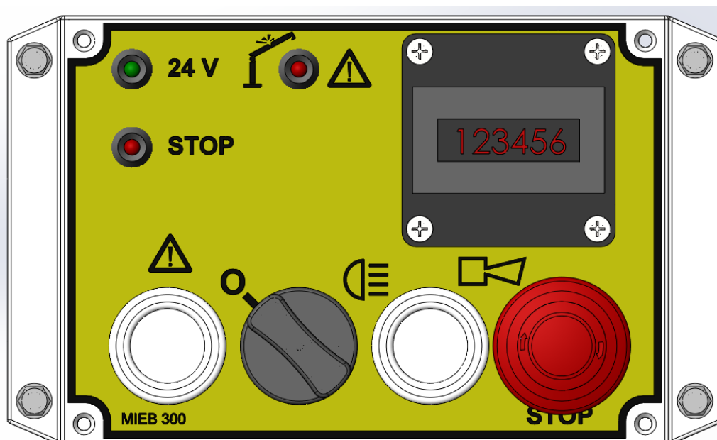
Рис.8: Блок индикации (пример)
