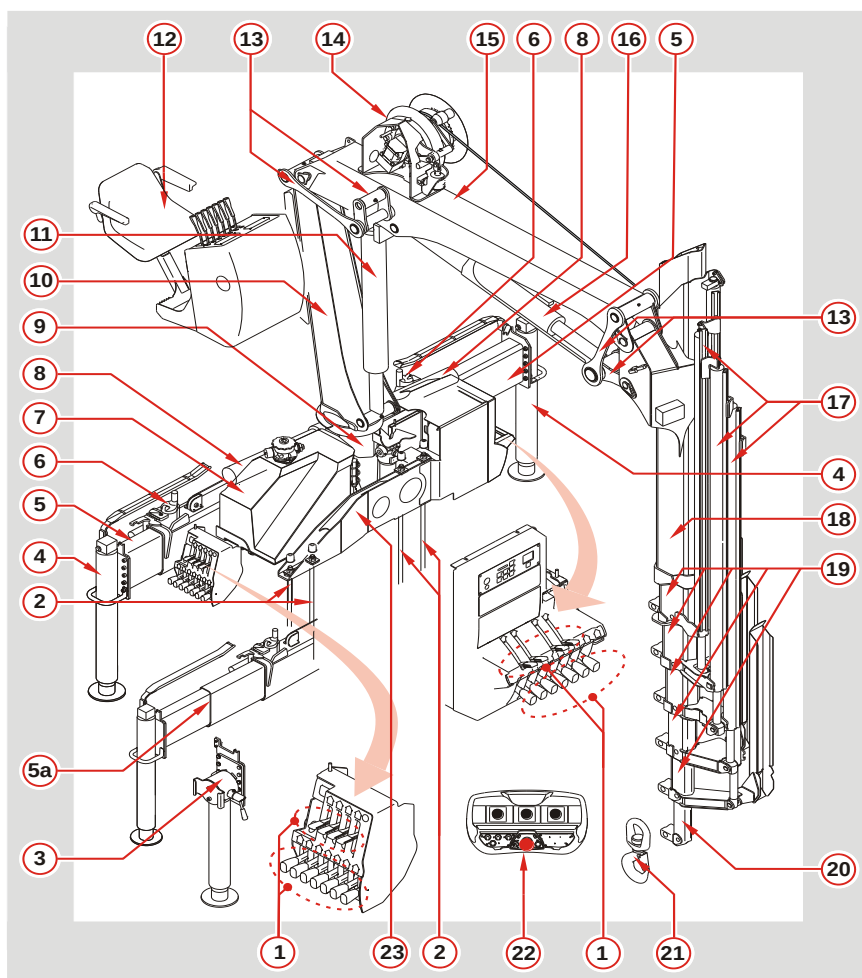
Рис.1: Устройство крановой установки (пример)
