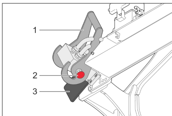
Рис.15: Быстроразъемное соединение для гидравлического оборудования
