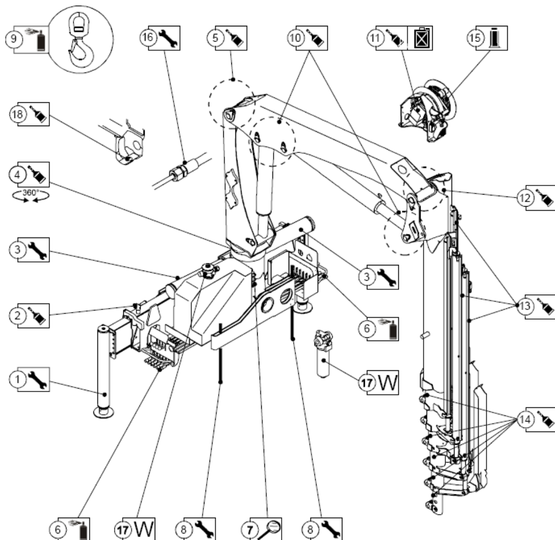
Рис.24: Схема обслуживания крановой установки
