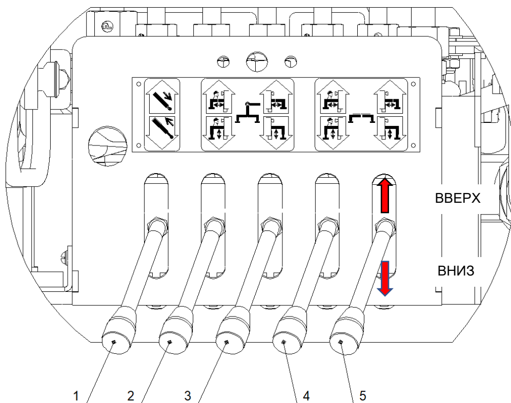
Рис.17: Панель управления со стороны гидрораспределителя аутригерами и опорными гидроцилиндрами КУ (пример)
